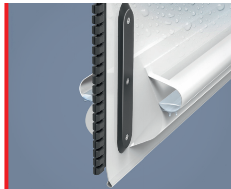
Sistema di drenaggio opzionale
